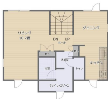
2階縮尺 1/150
